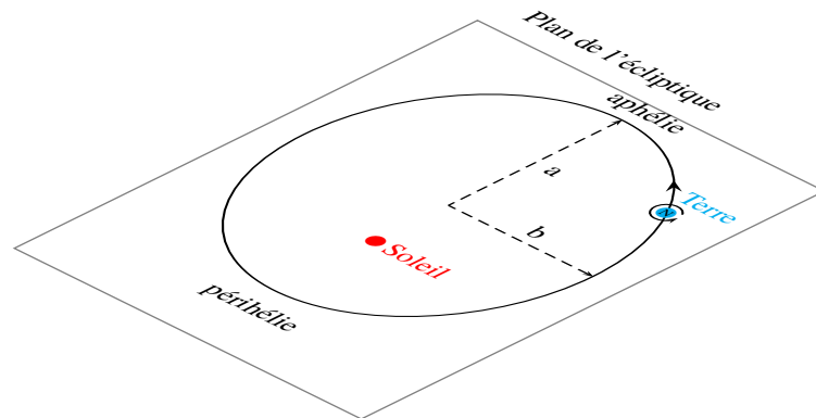
FIGURE 2 – Plan de l'écliptique
