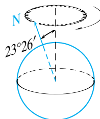
FIGURE 5 – Précession et Nutation
