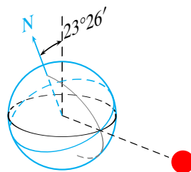
FIGURE 7 – Equinoxe d'automne dans l'hémisphère Nord
