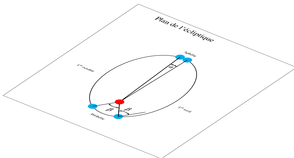
FIGURE 11 – Révolution de la Terre autour du Soleil
