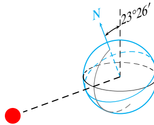
FIGURE 6 – Solstice d'été dans l'hémisphère Nord
