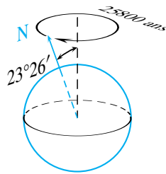
FIGURE 4 – Précession
